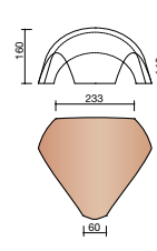
B000 5330 * Rencontre base poinçon 3 directions demi-rondes
