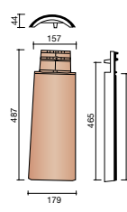
MK10 8010 Demi-tuile (2,6 au ml)
