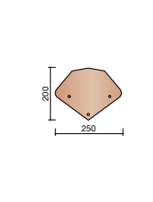
B000 2240 ● Écusson d'abergement Shed
