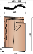
MK10 8100 Tuile de sous-faitage (4,1 au ml)
